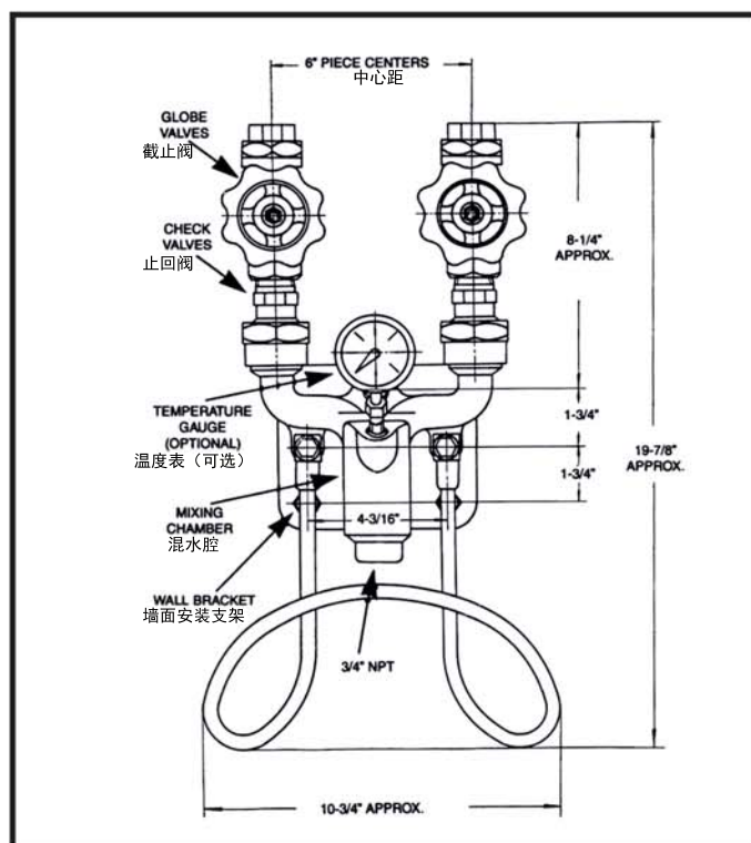
正视图
