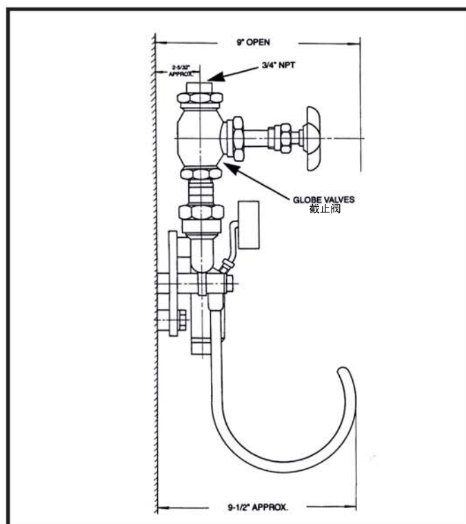
侧视图
