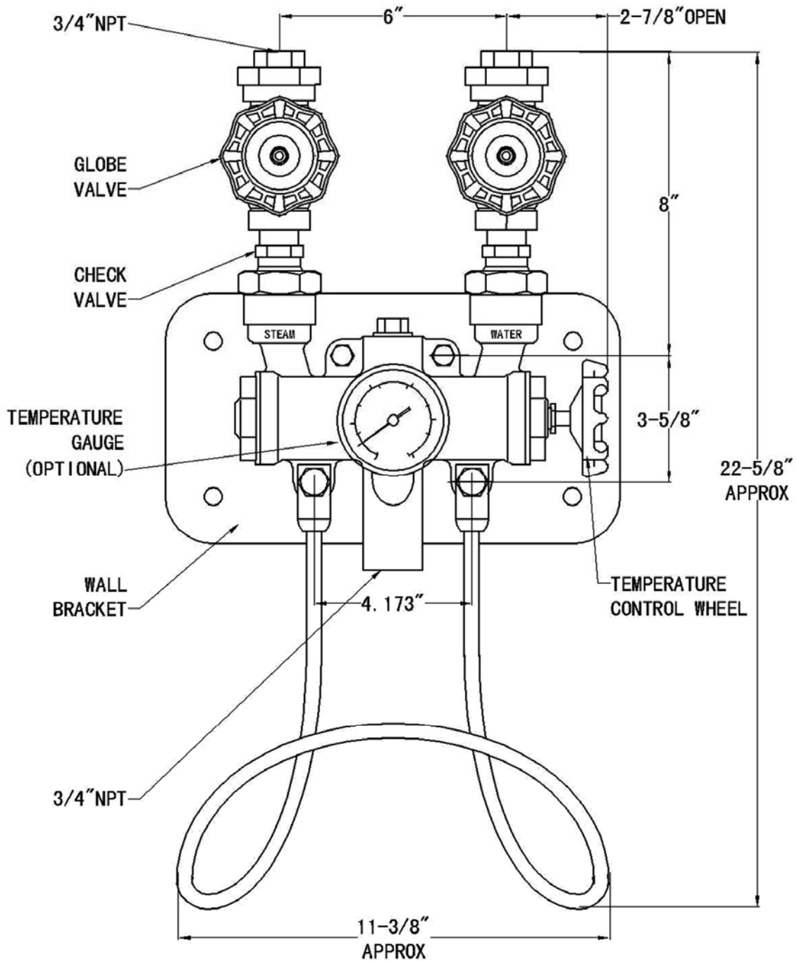
产品正视图
